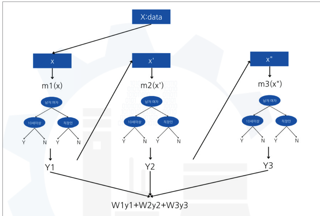
[그림 6] XGBoost 모델
