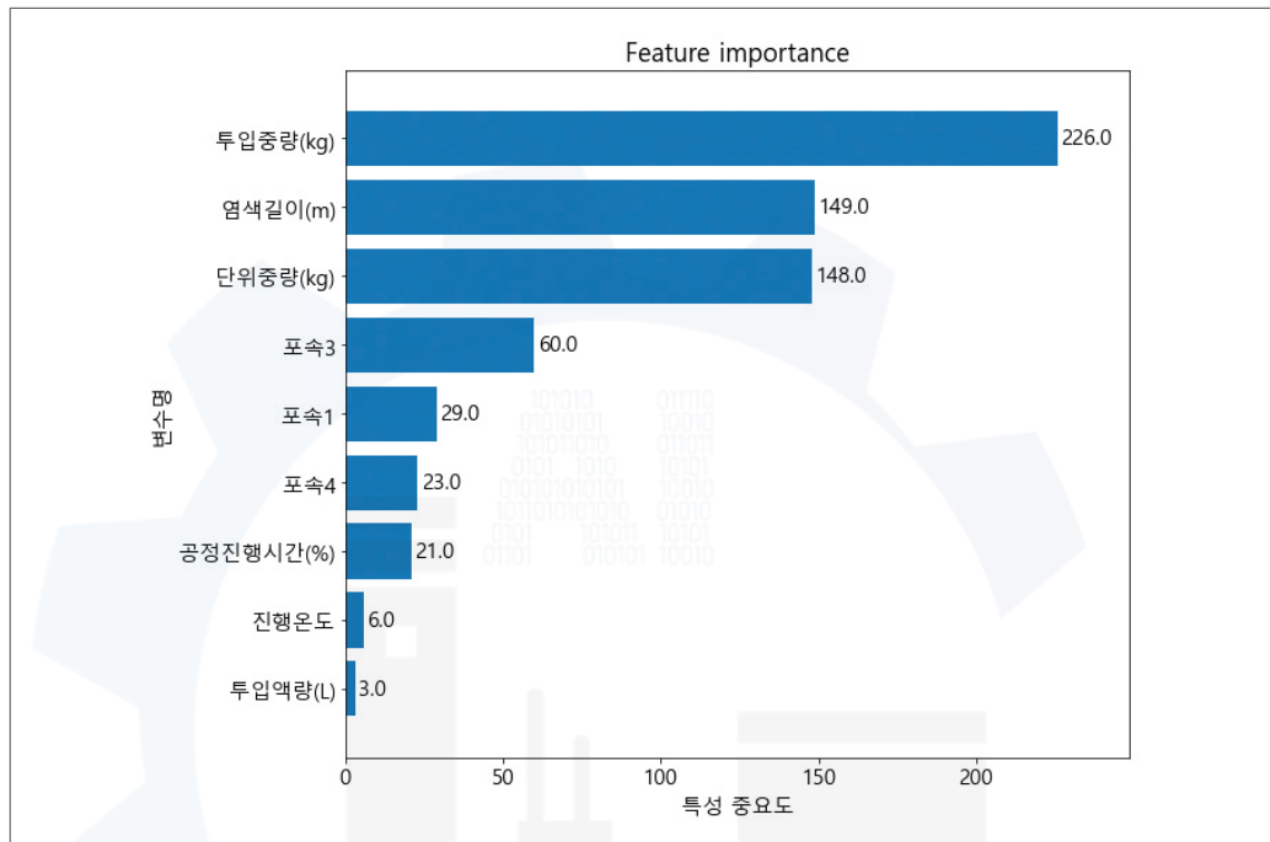
[코드 66] 특성 중요도
