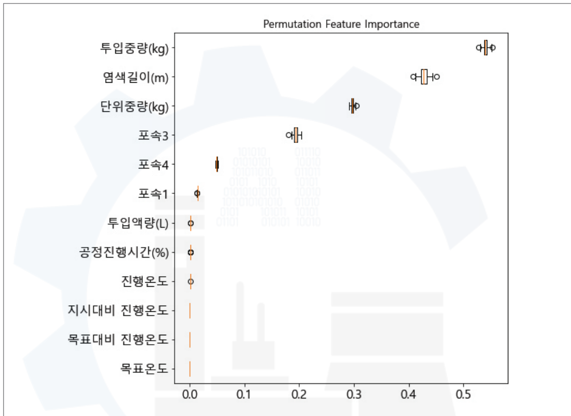
[코드 67] 순열 중요도
